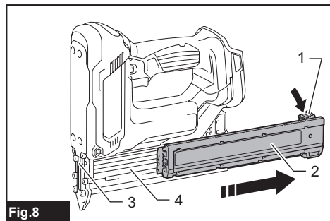
Fig. 8 ► 1. Palanca de bloqueo 2. Compuerta corrediza 3. Guía del tornillador 4. Cartucho
